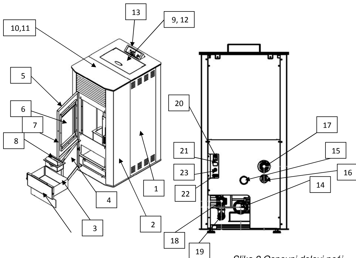
Slika 2 Osnovni delovi peći
